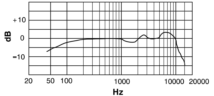
TYPISCHER FREQUENZGANG
