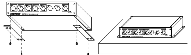
顶部安装
